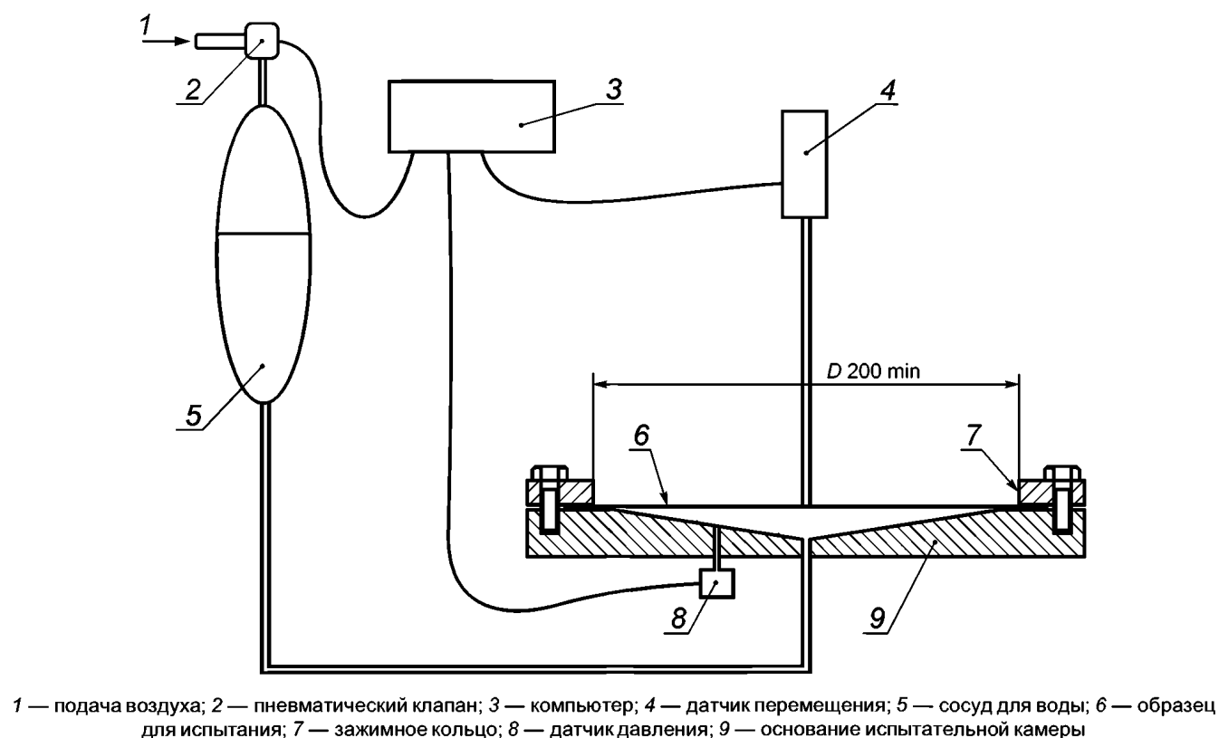
Рисунок ДВ.1 — Испытательная установка
